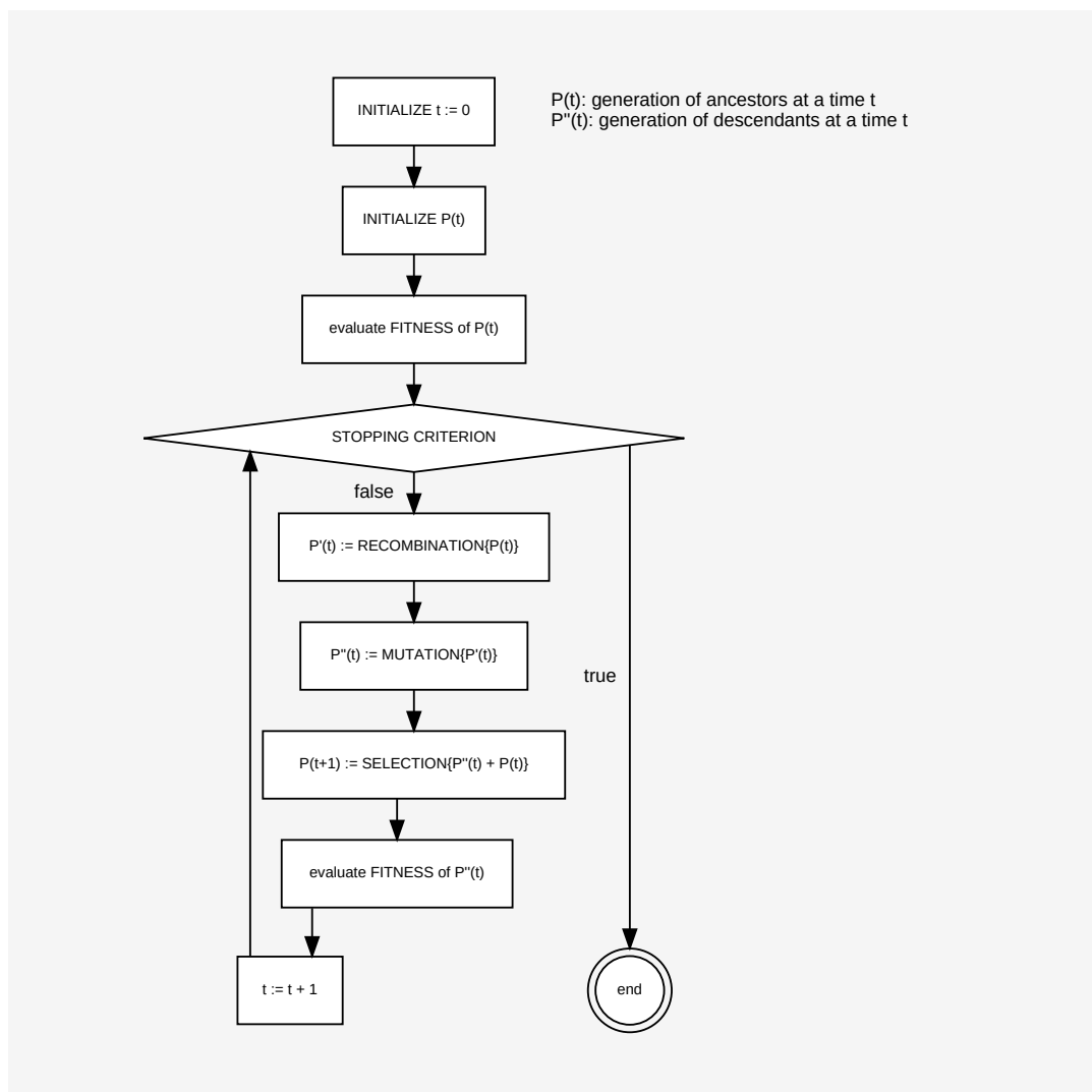
Figure 61.1. 遗传算法的结构
