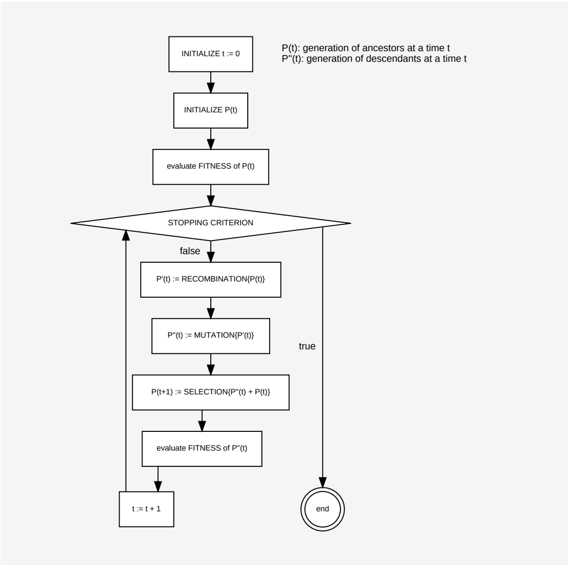
Figure 61.1. 遗传算法的结构
